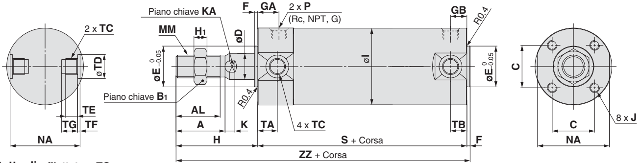
Dettaglio filettatura TC
