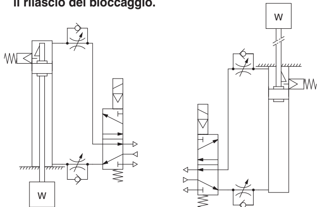
Bloccaggio su testata posteriore
