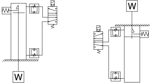
Bloccaggio su lato testata posteriore Bloccaggio su lato testata anteriore
