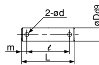
Perno snodo sferico Perno cerniera
