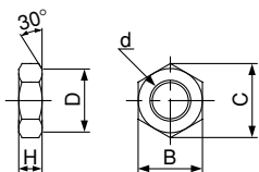
Dado estremità stelo (Standard)
