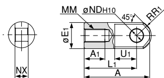
Snodo sferico
