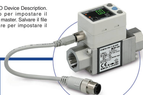
Dispositivo compatibile con IO-Link: flussostato digitale per acqua
