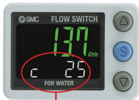
Indicazione temperatura
