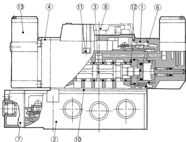
Bistabile 2 posizioni
