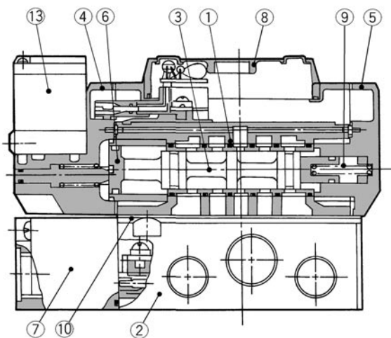
Monostabile 2 posizioni
