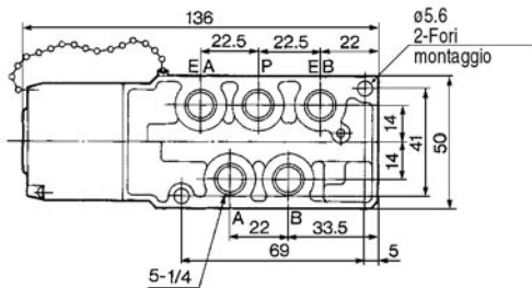
Attacchi inferiori
