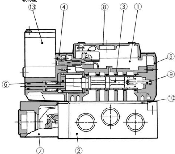
Monostabile 2 posizioni
