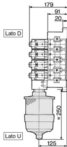
Montaggio lato U
