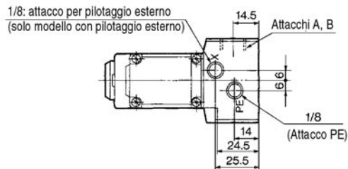
Attacchi inferiori
