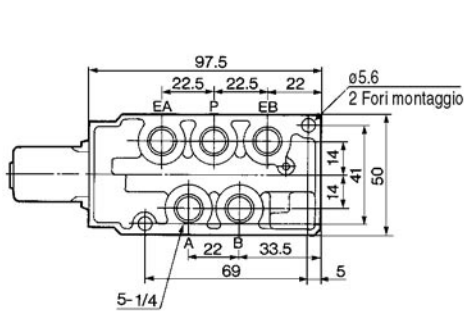
Attacchi inferiori
