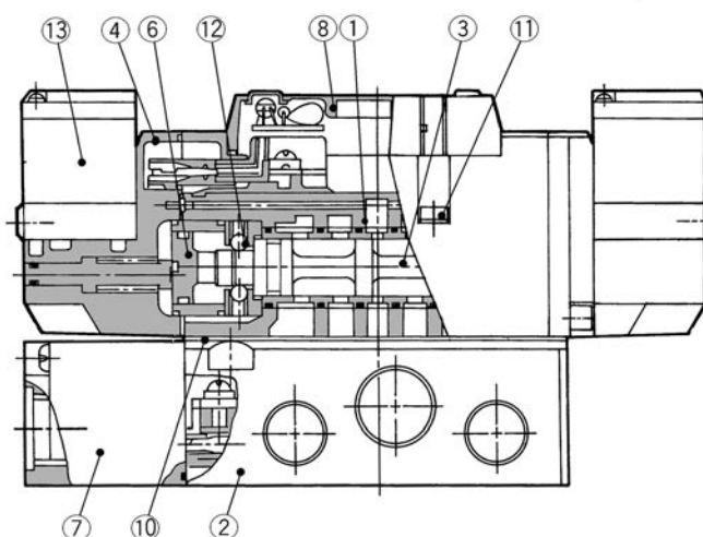
Bistabile 2 posizioni
